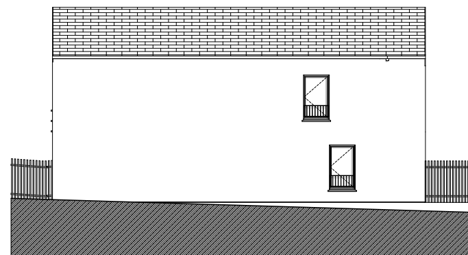
Façade Ouest
